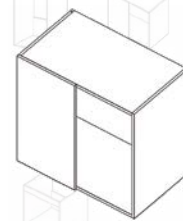
KTS009-L - korpus spodní rohový - rovný levý
