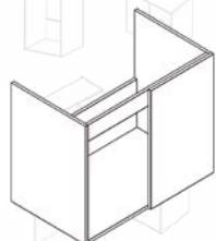
KTS006-P - korpus spodní rohový dřezový - rovný pravý
