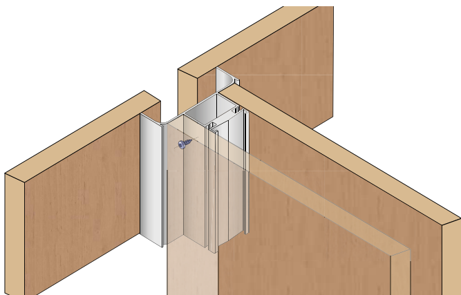
Profil vertikální C a J
