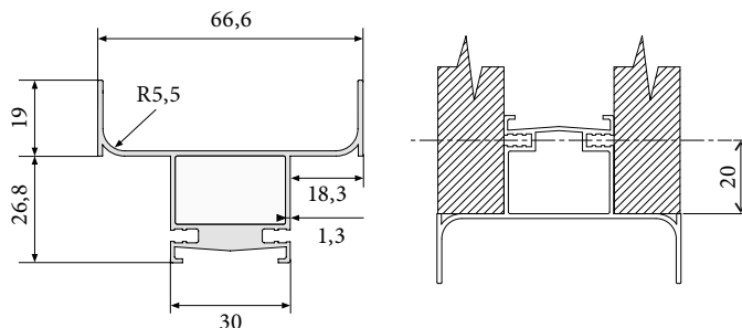
Profil vertikální C a J
