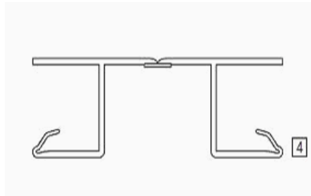
Spojka flexibilní (90-180 st.) 150mmk Soklové liště Rehau RAUBASE
