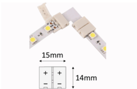
MO-LF10-L-D1 Konektor ve tvaru písmene L
