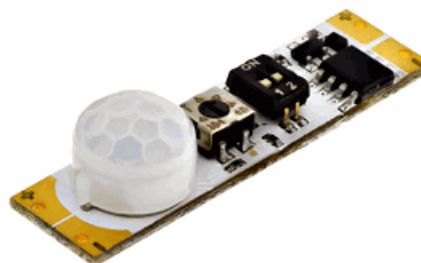
Vypínač do lišt PIR+SOUKRAK 45x10x7/9mm 7,5A 12V DC (90W) (C)
