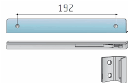
Slidix T25 tlumení k sadě S45 zadní/19C0T25Z/
