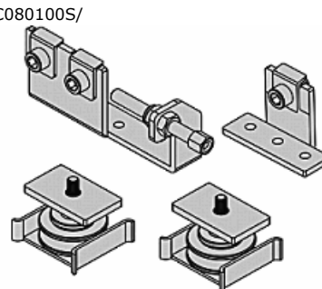
Sada pro synchronizaci 2 křídel S80/S100 /14C080100S/
