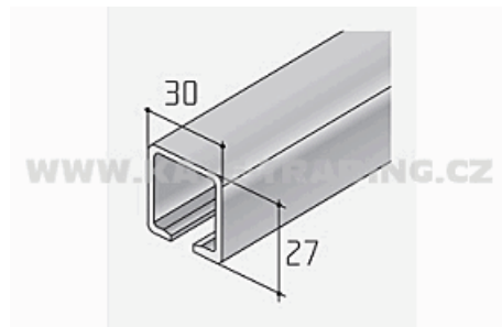
Profil S80 /S40 hliníkový /14C1S408N/ délka - 1m
