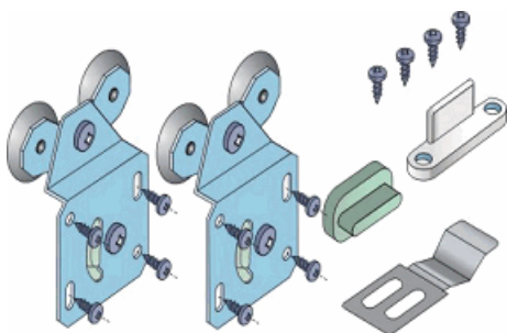
S42 SADA PREDNI /12C0S42P/
