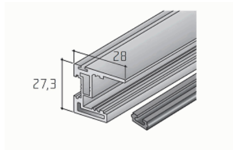
S45B madlo elox 2,7m /15D1S45B27/
