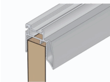
Profil Salu 11N 2,7 m stříbrný elox /17D1S11N27Bez /krycího profilu
