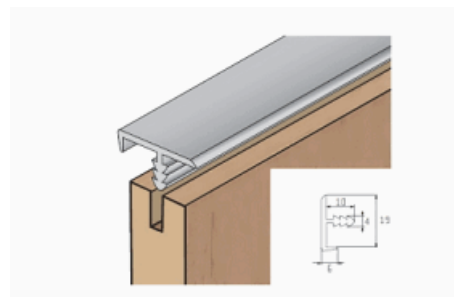
Narážecí hrana úchytná lišta S01 /1ND1NH01/ 1bm
