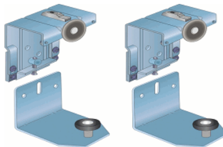
S45 sada na přední dveře /19C0S45P/
