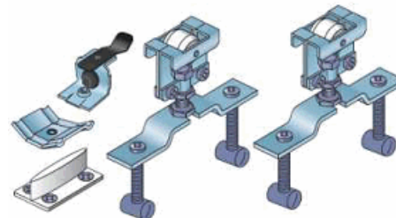
S 40H -Sada kování do 40 kg /14C0S40H/
