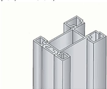
Profil boční S15 2.70m stříbrný elox-bez krycí profil/17D1MS1527/
