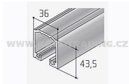
Profil pro kování S 100 ELOX /18D1S100/ 1bm
