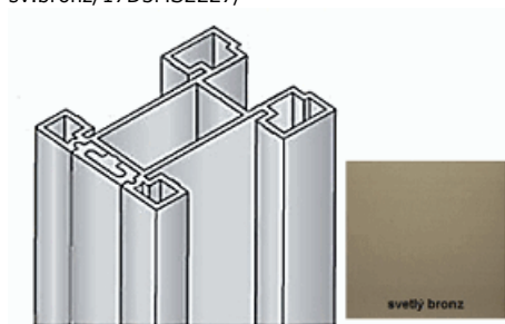
Profil boční S15 2.70m +krycí profil sv.bronz/17D3MS2227/
