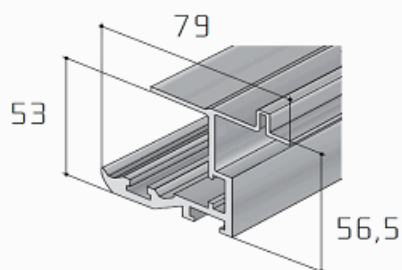
S45 horní profil /19D1S45H/ délka 1bm
