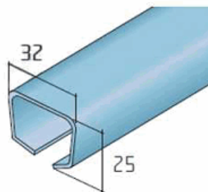
Profil S40/S80 ocelový profil cena za 1bm /14C9S408/
