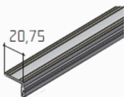
S40SD – dolní profil /15A0FPKL/ délka 2m
