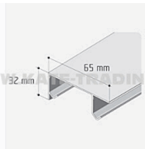
Profil S 30 dvojitý /12D2DVOJ/ délka 1bm
