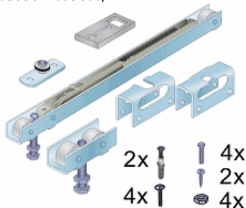
Sada kování S80Frame pro S65 SC C60 /14C0S8SCFR65SC60/
