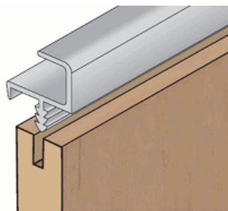
Profil S 02 ELOX 1bm /2 a 3 m /1ND1NH02/
