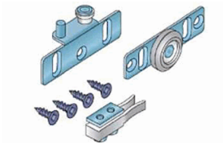
Sada kování S 27AL pro Hliníkové rámy úzké/13C02737/
